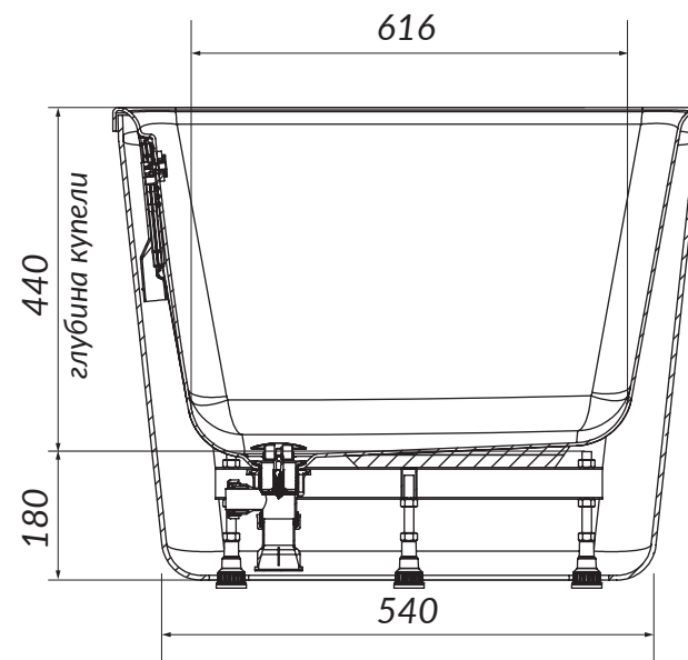
поперечный разрез ванны
