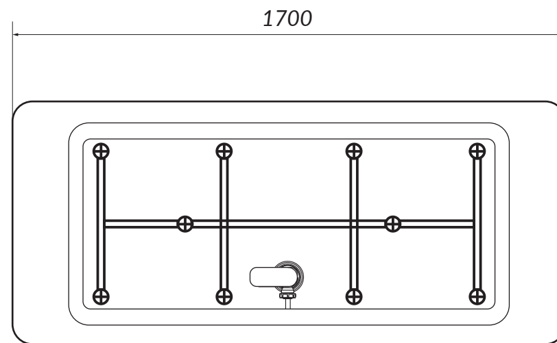
схема расположения опор (вид снизу)
